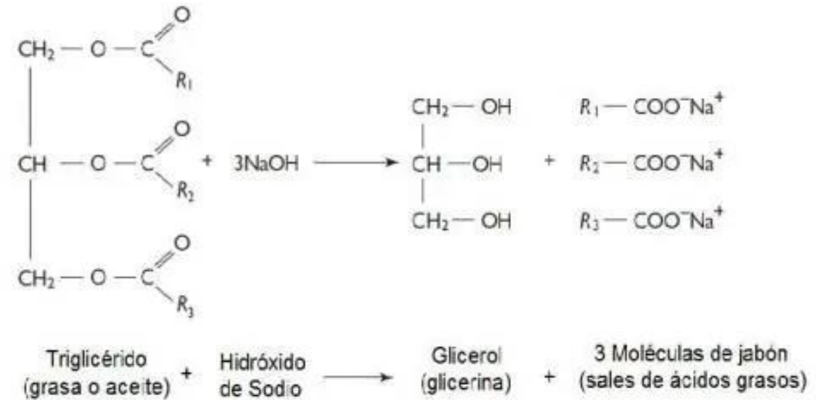
Figura 3. Saponificación de un triglicérido.
