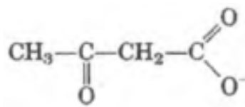
Acetoacetato
