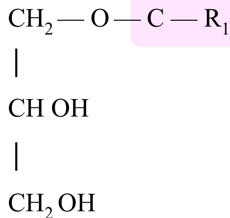
1-Monoacilglicérido
