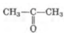
Acetona
