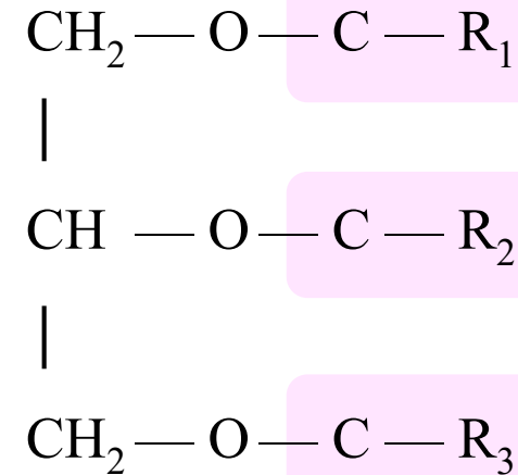
Triacilglicérido Grasas neutras
