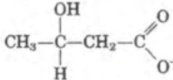
D-β-Hidroxibutirato
