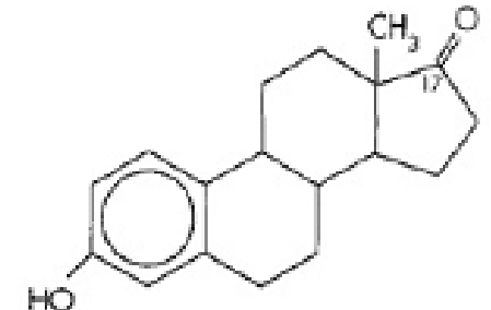
Estrona
