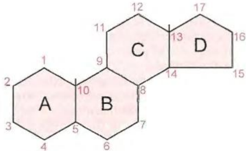
Fig. 5-14. Ciclopentanoperhidrofenantreno.
