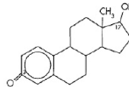
Estradiol
