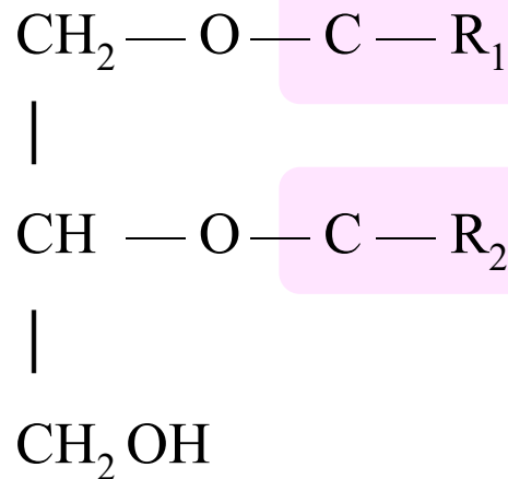
1,2-Diacilglicérido
