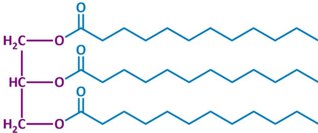
Estructura ejemplo de un TAG que forma grasas
