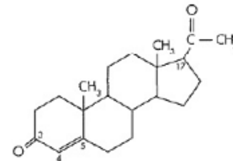
Progesterona
