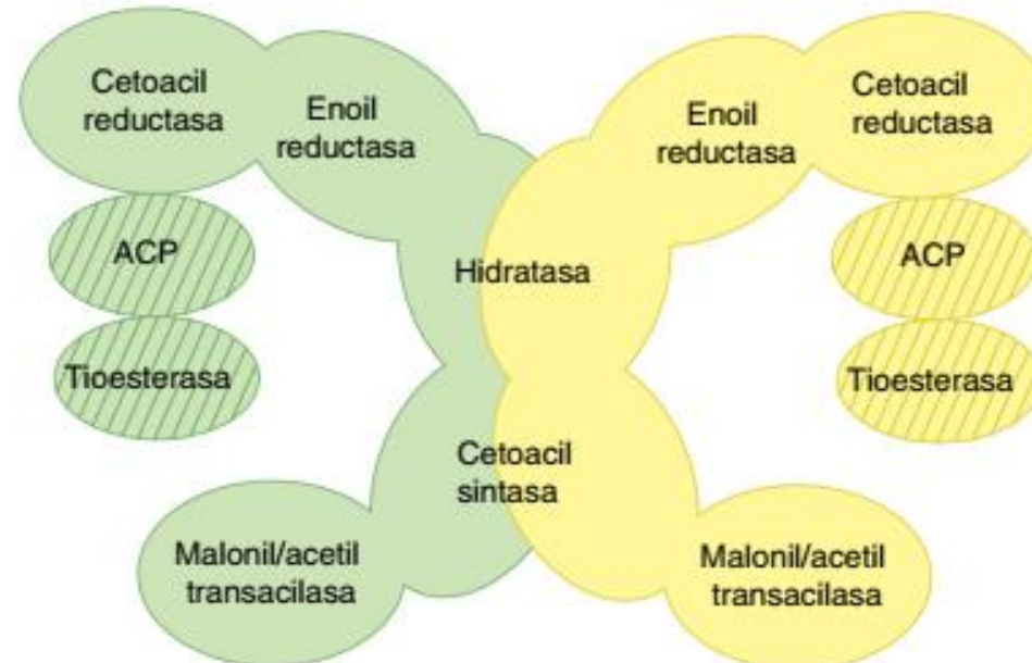
Homodímero de ácido graso sintasa
