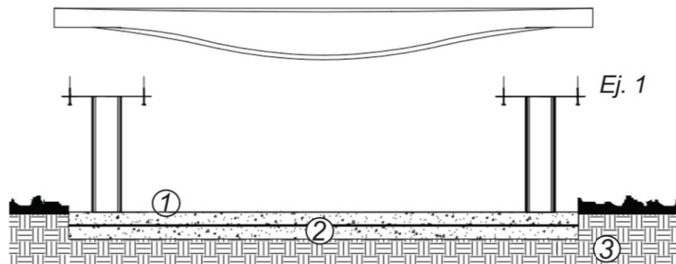
Vista 2 - Escala 1:...
