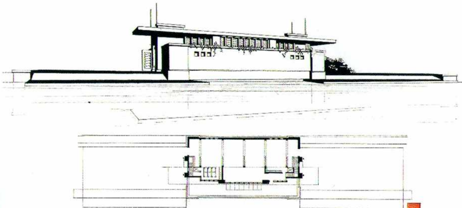
Ilustración página 4 ►Casa guardabotes rio Yahara, Madison (Wisconsin), 1905, perspectiva y planta
